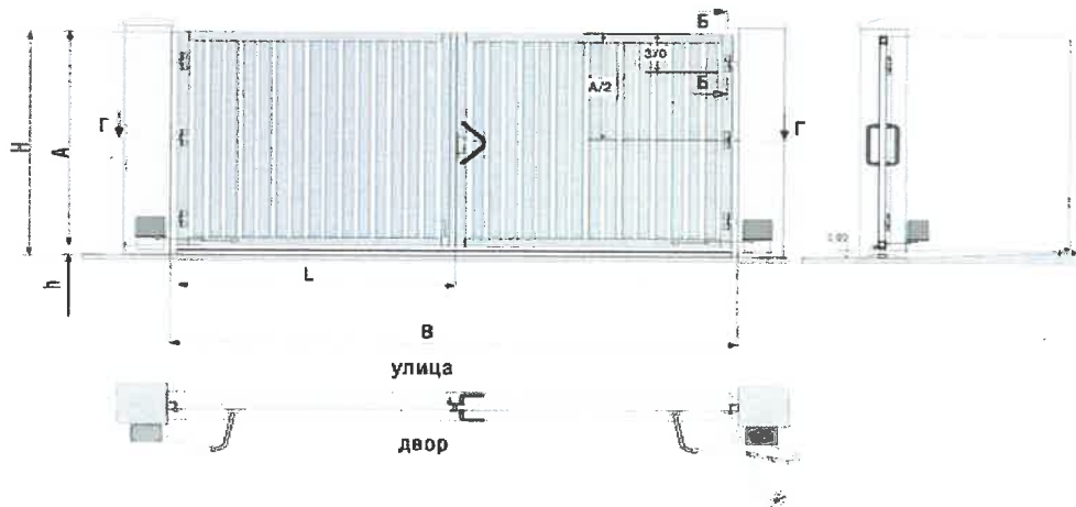
Внешний вид ограждающего устройства (габариты: 3890x1800мм)
